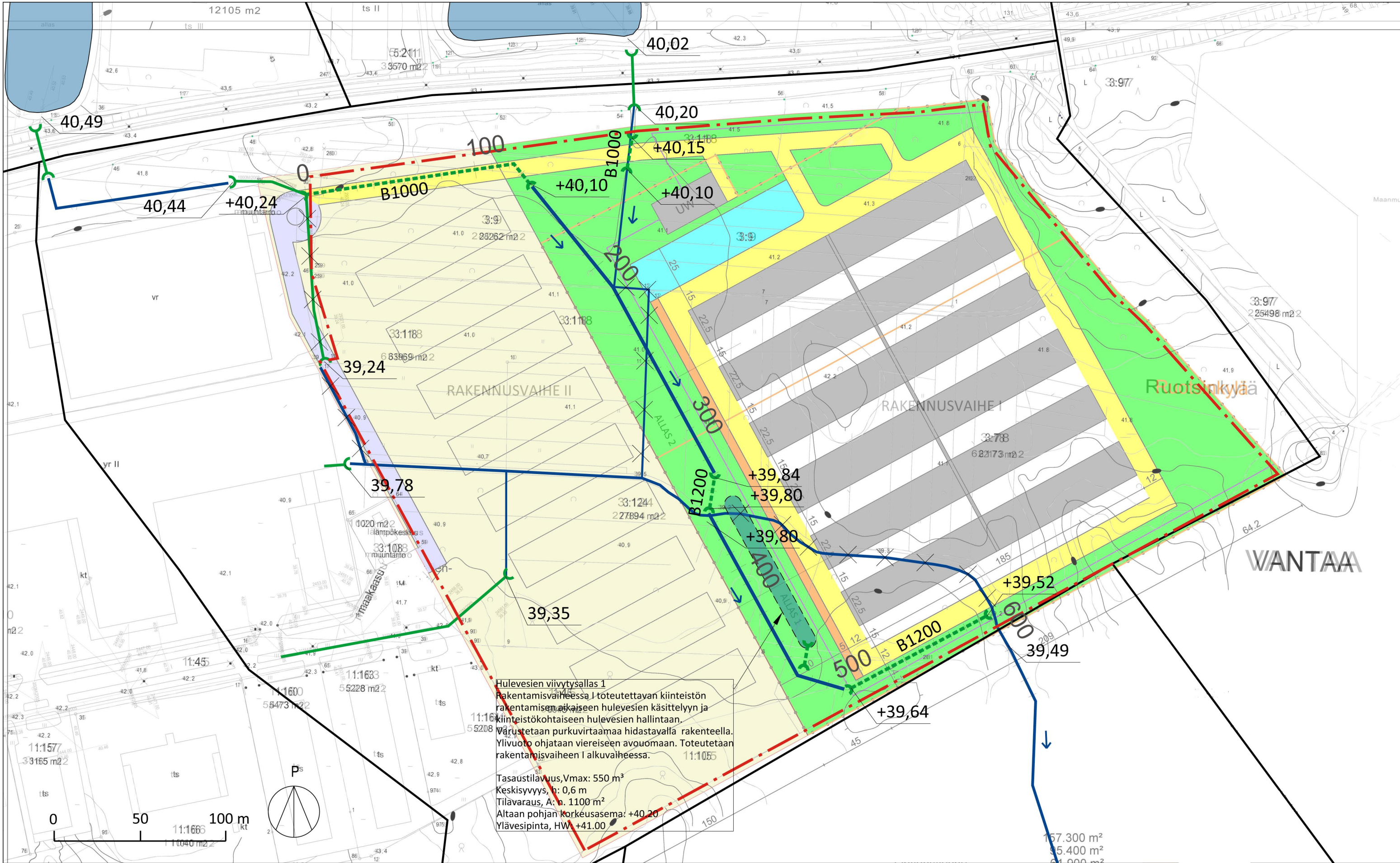
KULOMÄENTIEN HULEVESISELVITYS LIITE 1. HULEVESIEN HALLINTASUUNNITELMA, TOTEUTUSVAIHE I, 1:2 000 (A3) 9.6.2015 A.J.Koskenniemi
