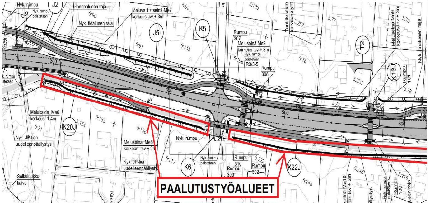
Kuva 1, paalutustyöalueet
